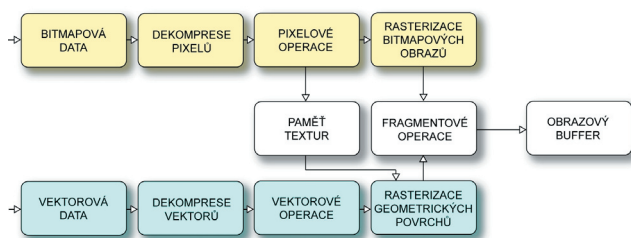
Obr.3: Zřetěžený proces tvorby obrazu systémem OpenGL
