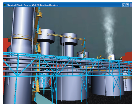
Obr.6: Při jednopřechodovém vykreslování maximálně využijeme „hrubý“ výkon grafické karty a nejvíce šetříme výkonem CPU
